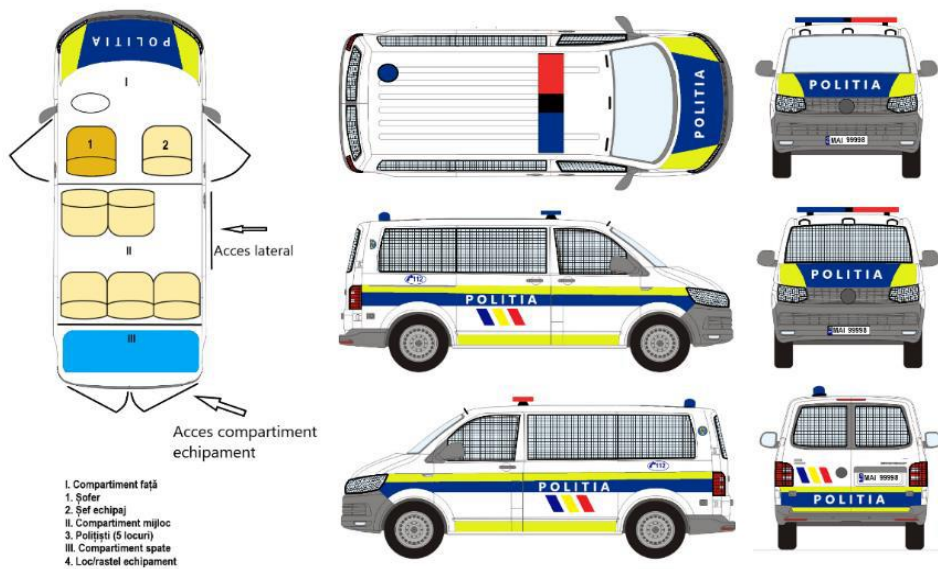
SCHIȚĂ MODEL "B" AUTOSPECIALĂ DE TRANSPORT ȘI INTERVENȚIE 6+1 6 LOCURI POLIȚIȘTI
